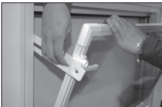
2. Zum Herausnehmen des Kippflügels die Schere leicht auseinanderziehen und über den Führungsstift drücken.
