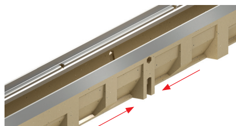
T-Verbindung (2 x 90°) über die seitlich geöffneten Vorformungen (beidseitig) am 0,5 m-Element
