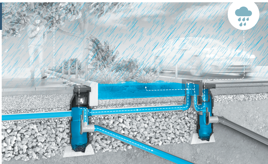
Figura 3: Il corpo della città di spugna è saturo - tracimazione facoltativa nella fognatura
