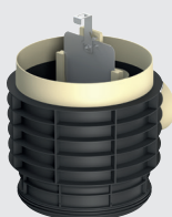
Sezione intermedia con scarico DN/OD 160 incl. cursore e troppopieno
