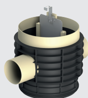
Sezione intermedia con ingresso e uscita DN/OD 160 incl. cursore e troppopieno
