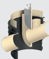
Sezione intermedia con ingresso e uscita DN/OD 160 incl. cursore e troppopieno
