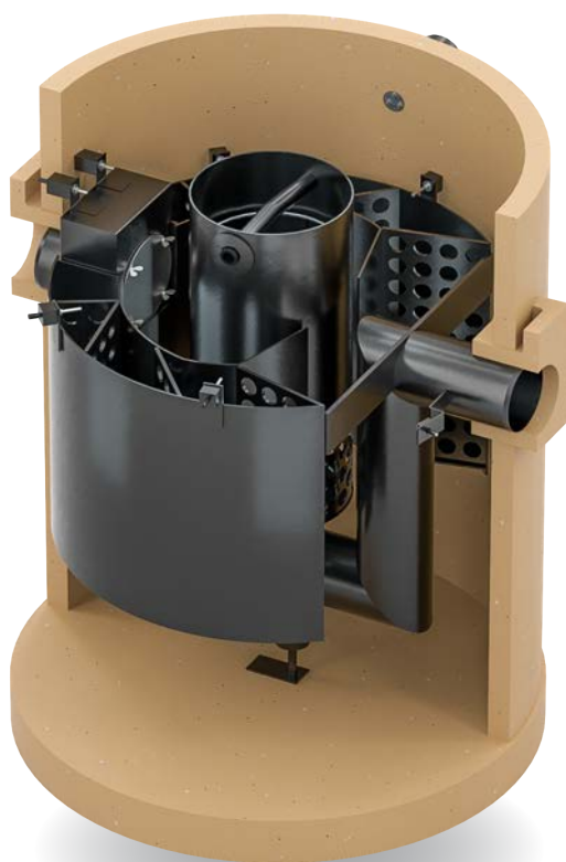
ACO Oleosmart in calcestruzzo polimerico
