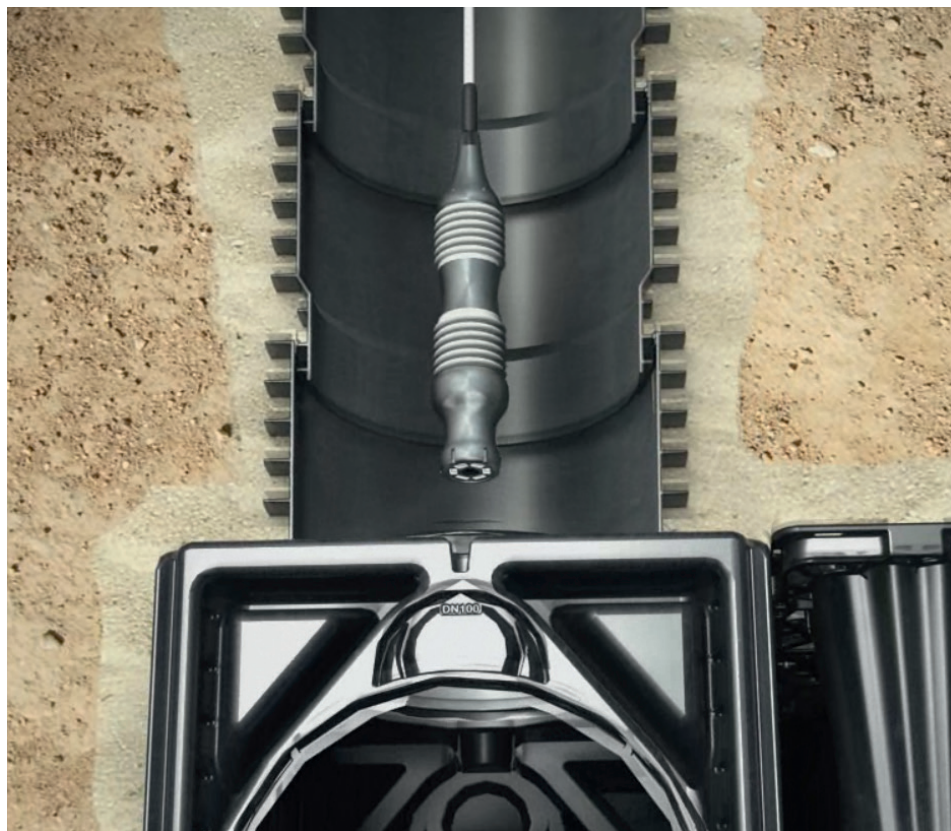
La telecamera di ispezione viene inserita verticalmente nel sistema di infiltrazione attraverso le parti superiori di ACO Stormbrixx e le parti inferiori o intermedie del pozzetto.
