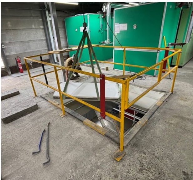
Montage ACO Sonderschachtabdeckung
