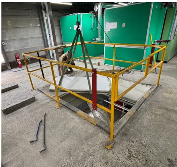
Montage du couvercle spécial ACO
