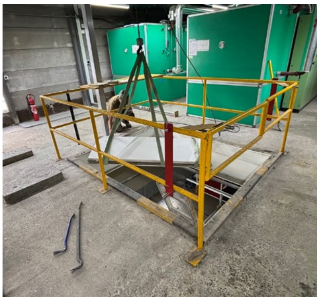
Montaggio del chiusino speciale ACO
