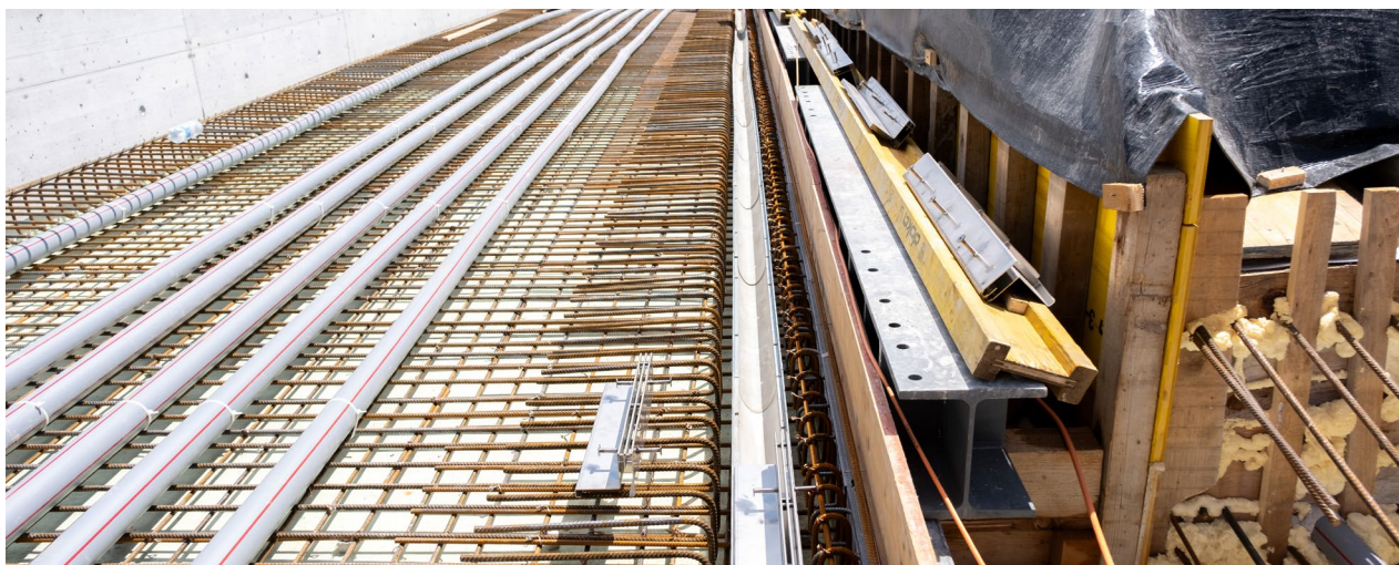
Installation des caniveaux ACO NEXITE® avec rehausse à double fente en acier inoxydable V4A avec boulons en acier inoxydable
