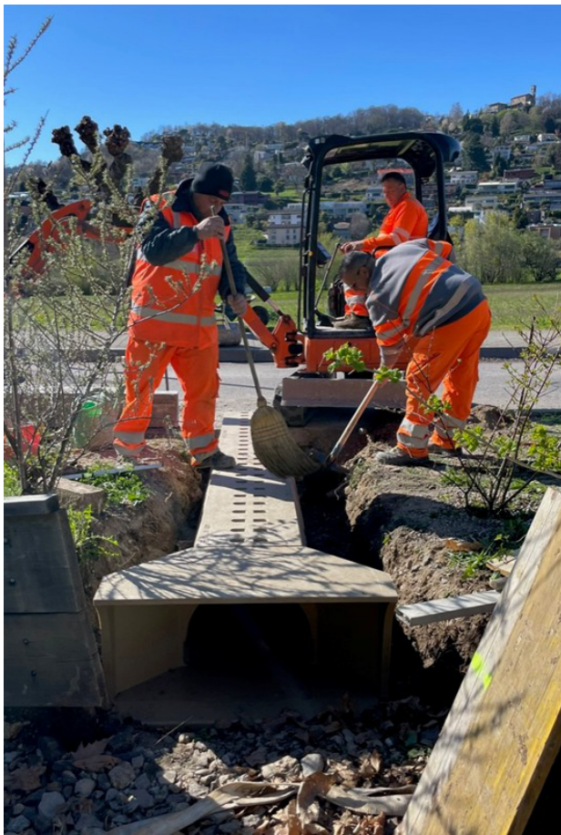
Trichterförmiger Eingang in den ACO Amphibien-Tunnel
