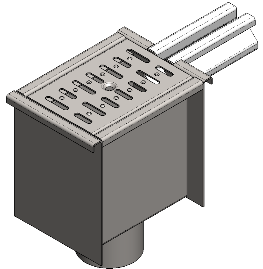
Anschlussbeispiel: Schlitzrinne
