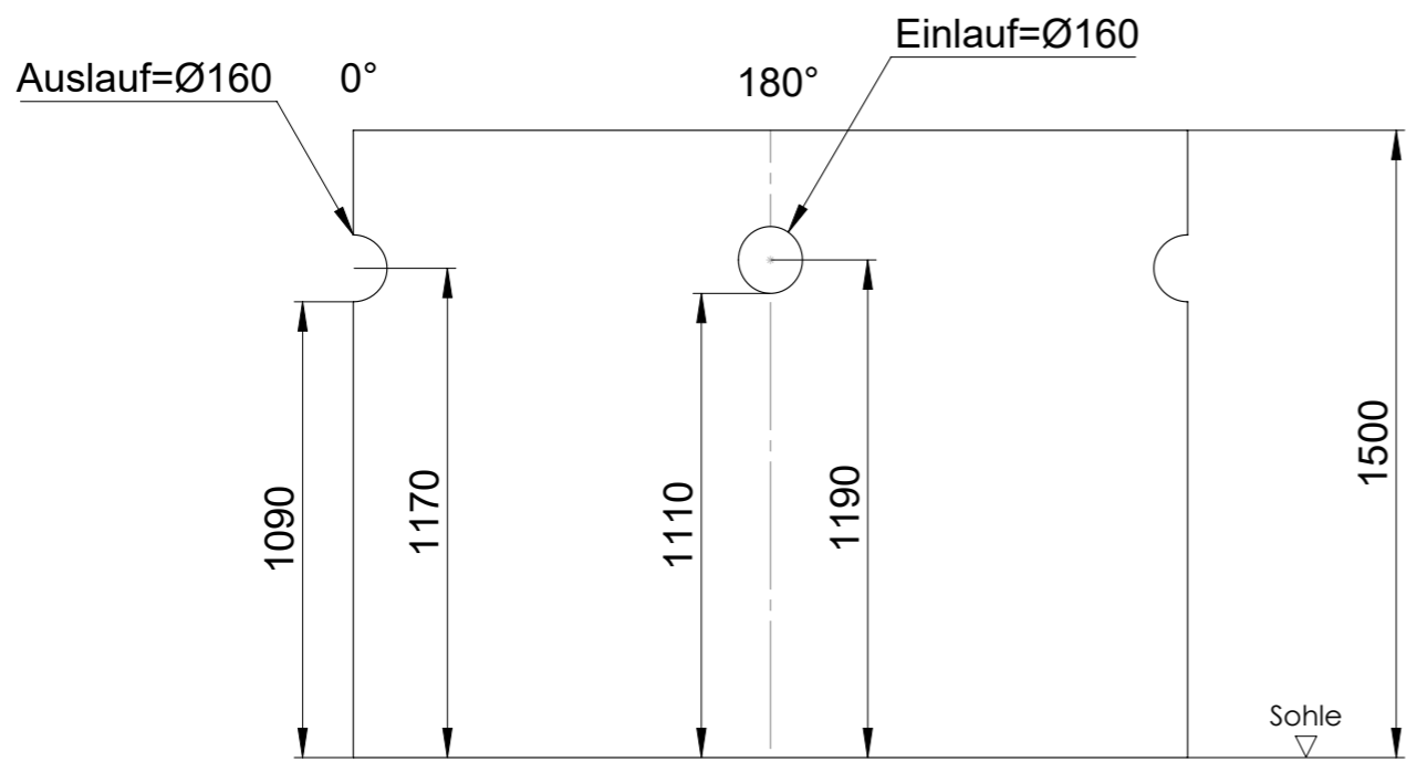
Abwicklung (1:20)
