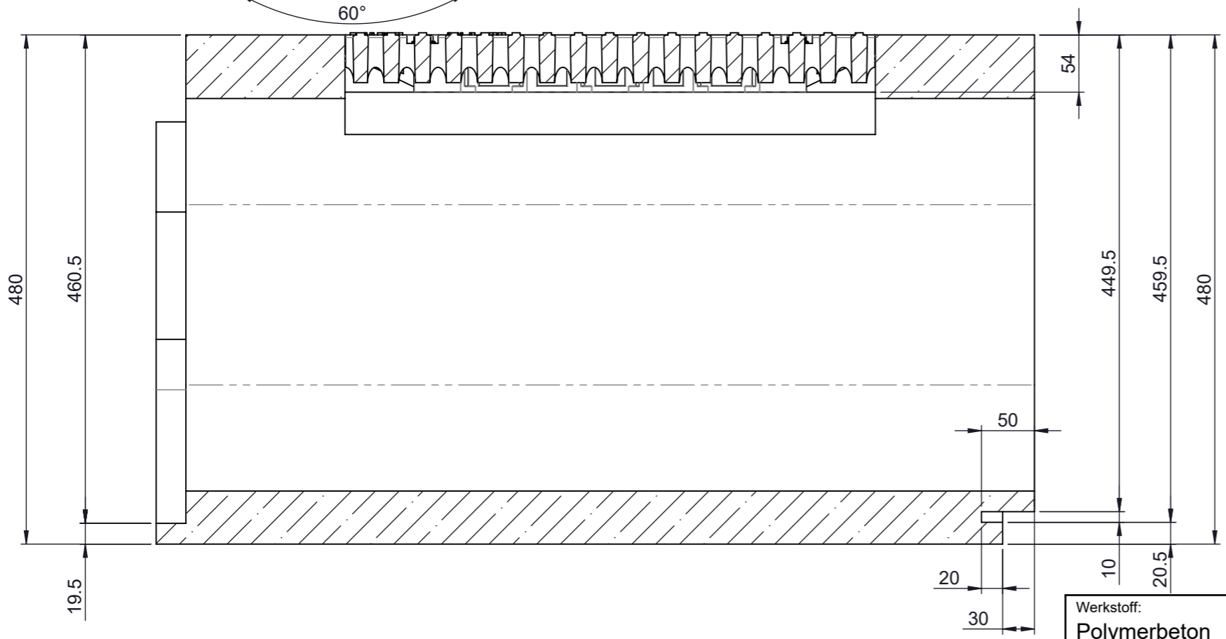
SCHNITT A-A MAßSTAB 1 : 5
