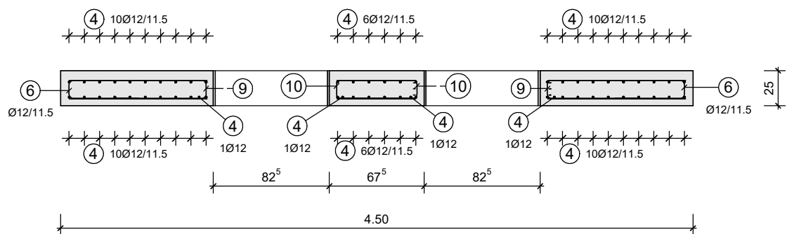
Schnitt 3 - 3
