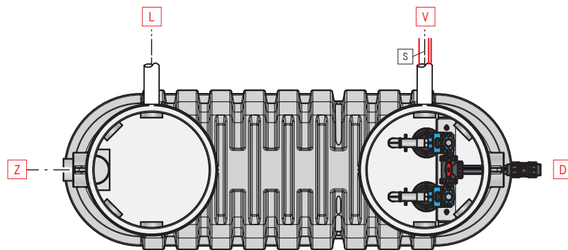
Abbildung: Anlage_Draufsicht
