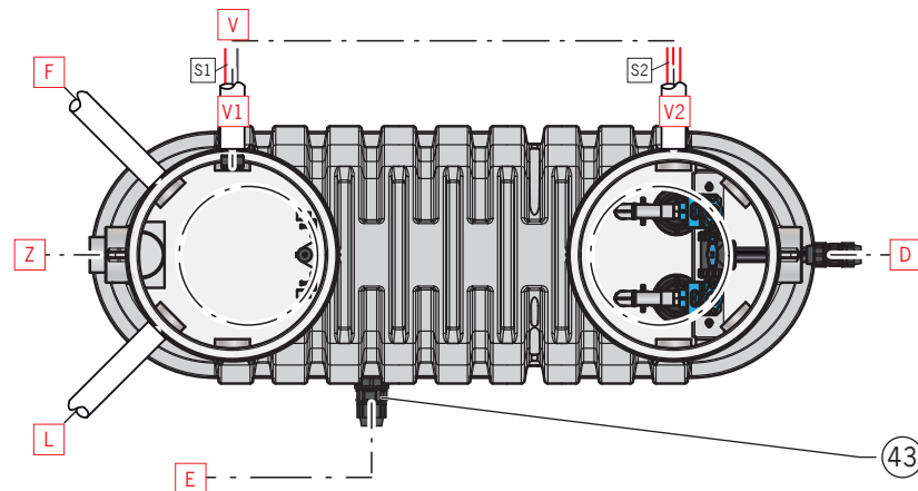
Abbildung: Anlage_Draufsicht
