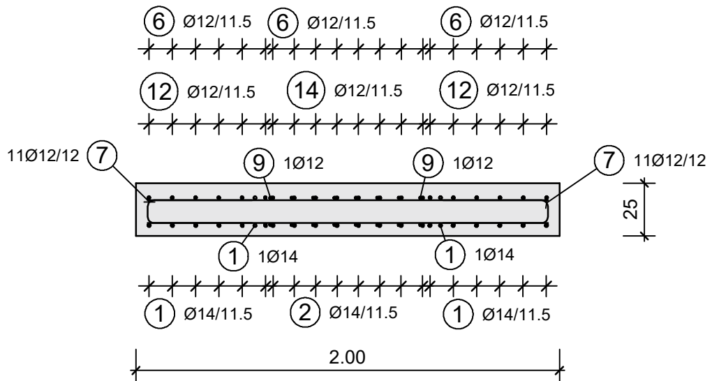
Schnitt 1 - 1
