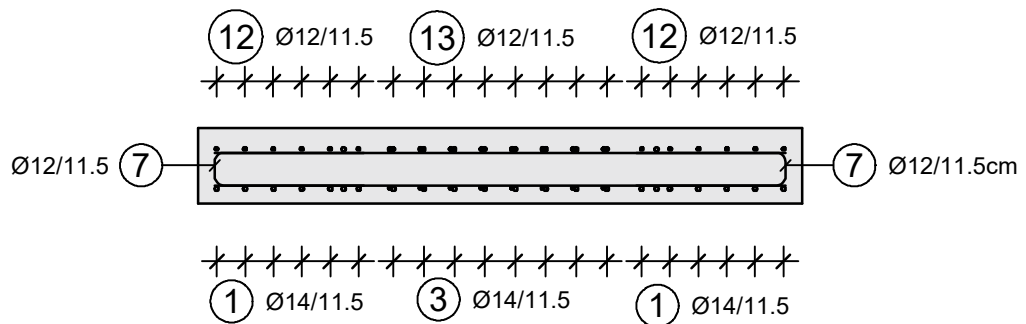
Schnitt 2 - 2
