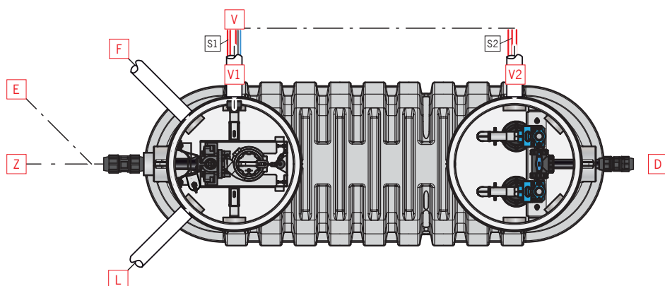
Abbildung: Anlage_Draufsicht
