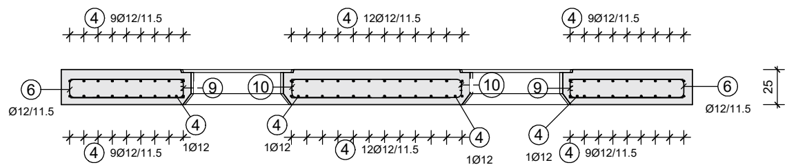
Schnitt 3 - 3
