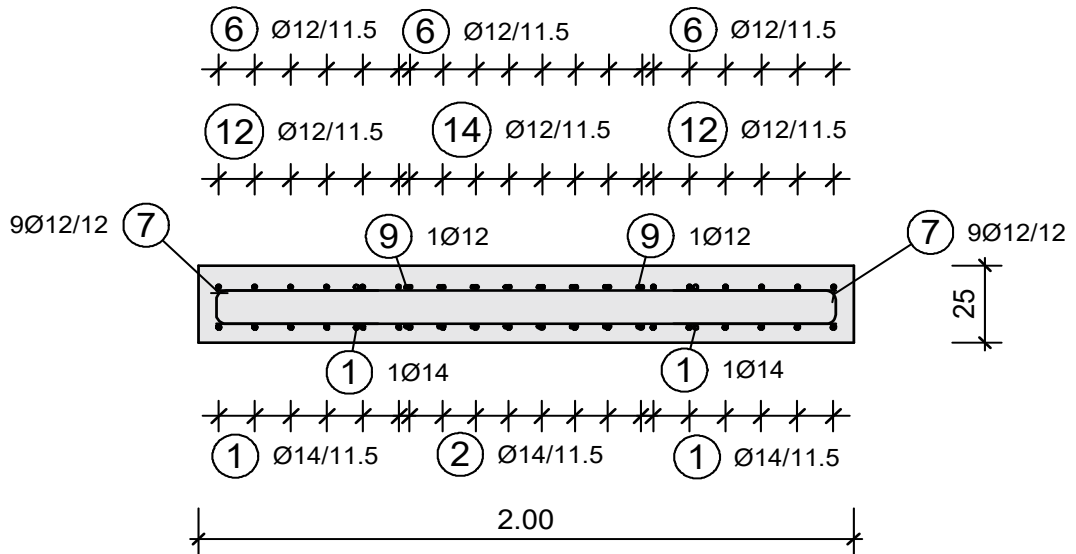
Schnitt 1 - 1
