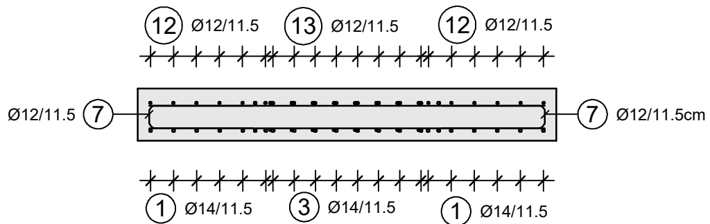
Schnitt 2 - 2
