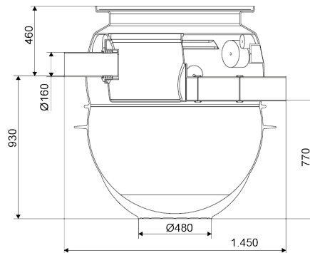
Parte inferiore del pozzo di circolazione (fase di costruzione #1)
